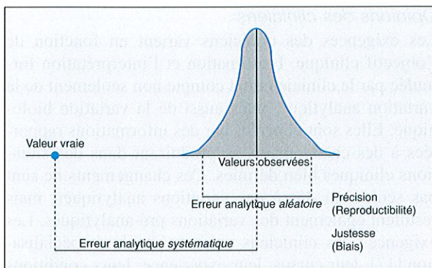
Figure 1. Schéma illustrant le concept d'incertitude des mesures.
